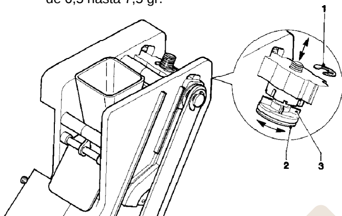
Fig. 13 1 - Anillo elástico 2 - Piston superior 3 - Aletas de referencia
