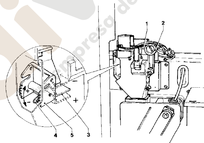
Fig. 14 1 - Molinillo 2 - Manecilla de ajuste del molido 3 - Regulador de dosis 4 - Palanca de regulación dosis 5 - Muescas de referencia
