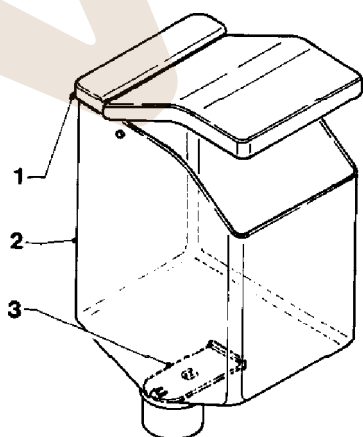
1 - Tapa 2 - Contenedor de café 3 - Cierre
