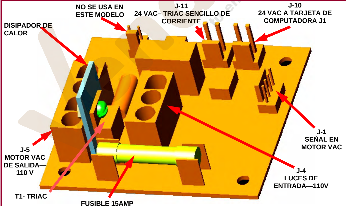
Fig. 22 (Tarjeta TRIAC)
