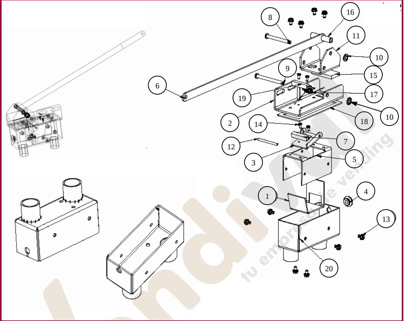
Fig. 29 (Ensamble de la caja de válvulas)
